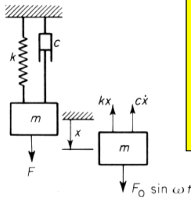
圖 1. 簡諧振動系統示意圖
